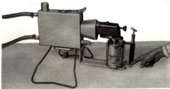
Bild 9. Blåslampan placerad på motorvärmaren
