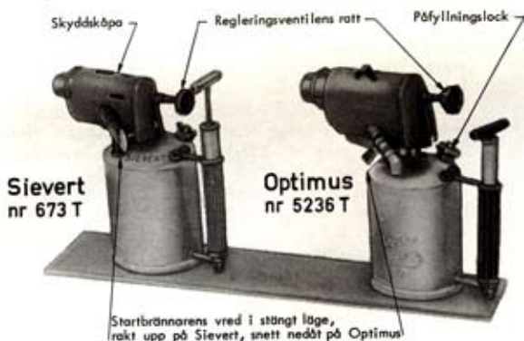
Bild 4. Blåslampor till motorvärmare 271
